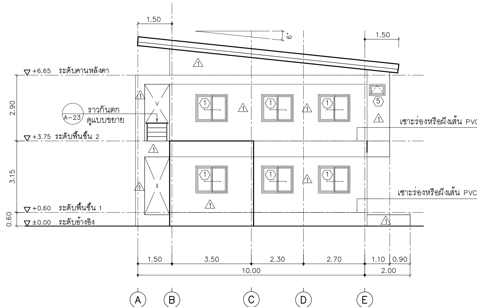
รูปด้าน 4
