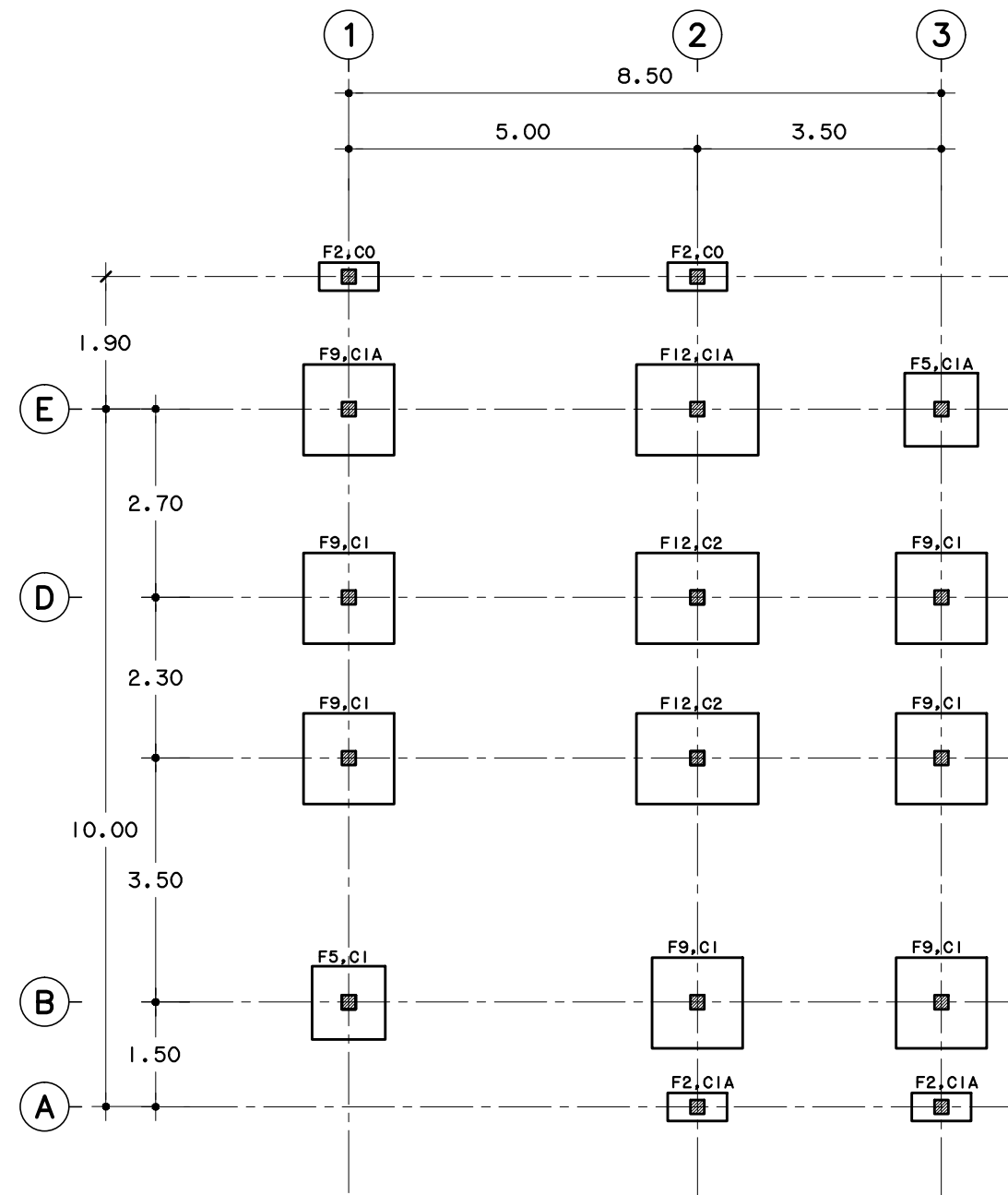
แปลนฐานรากเสาเข็ม มาตรฐาน 1:100
