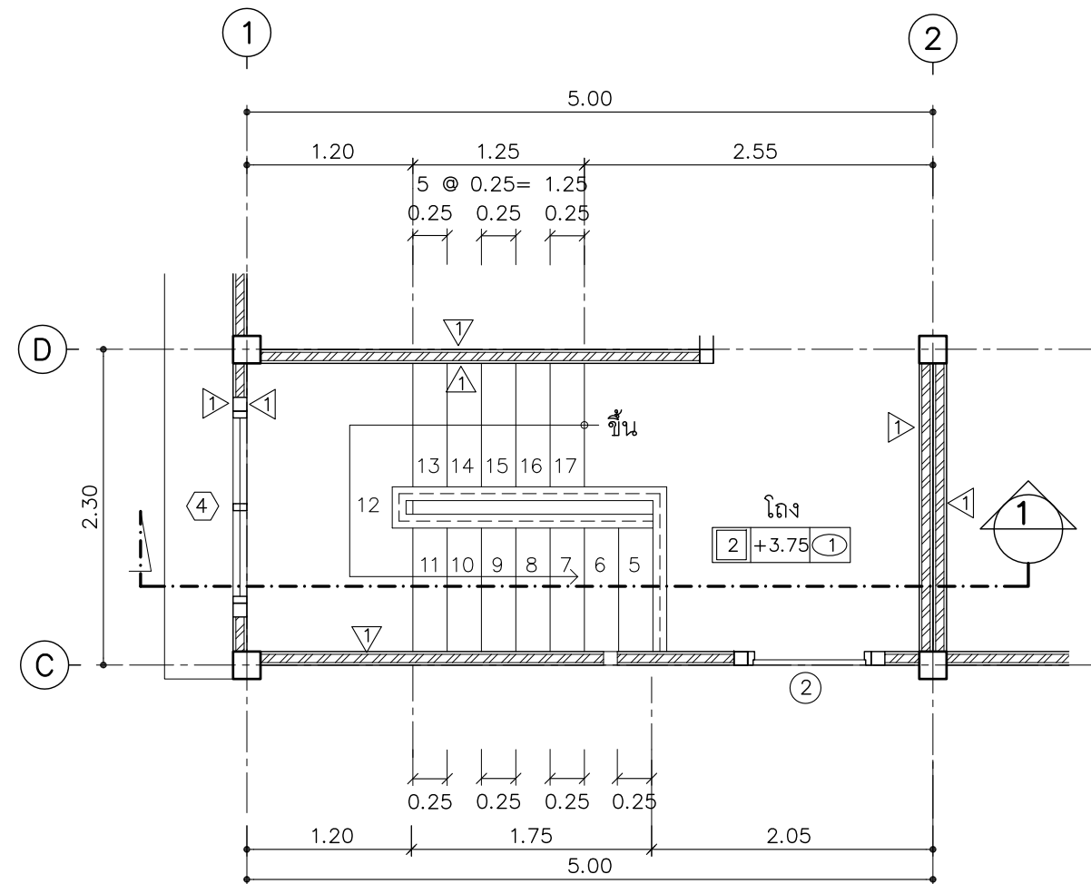
แปลนชั้น 2 บันได ST.3
