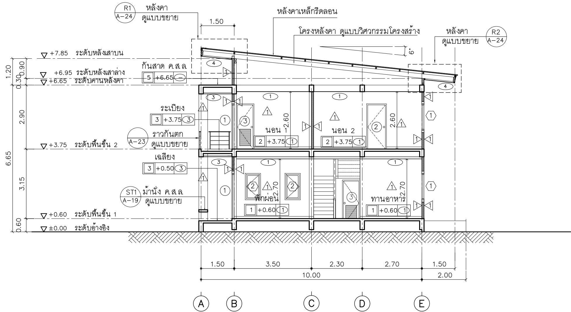
รูปตัด 2 มาตราส่วน
