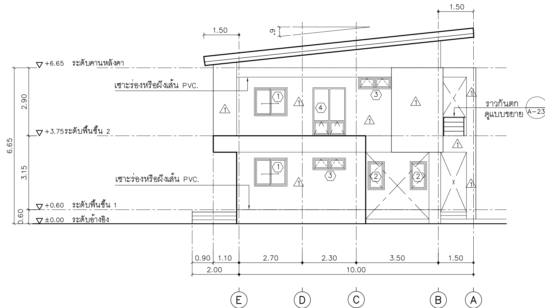
รูปด้าน 2
