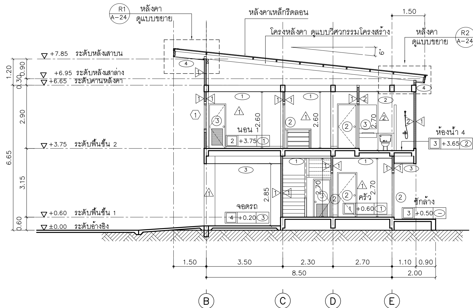
รูปตัด 3 มาตราส่วน 1 : 100
