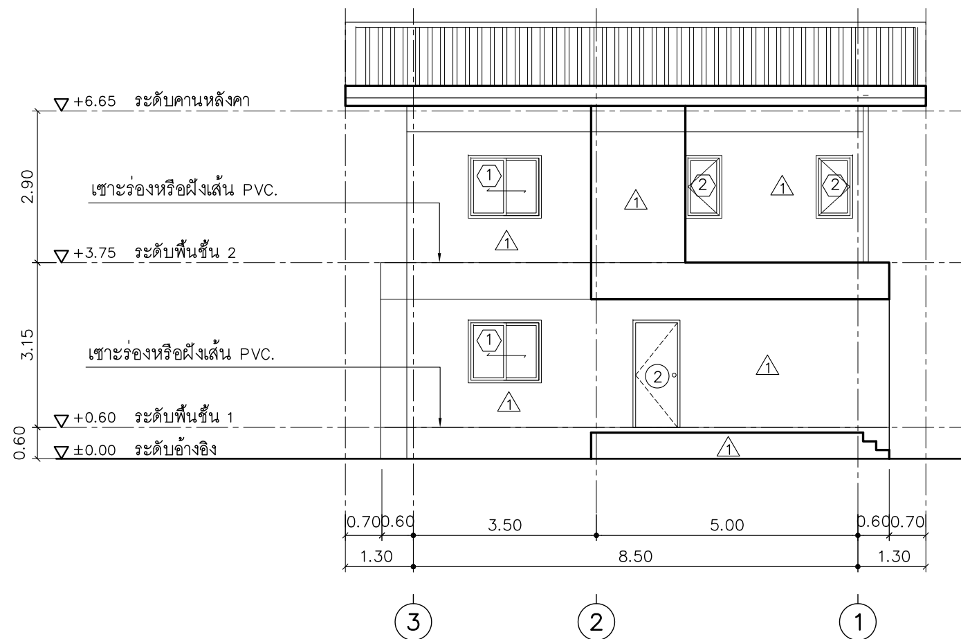
รูปด้าน 3
