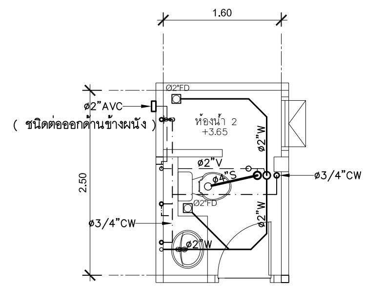
แปลนระบบสุขาภิบาลห้องน้ำ 3 มาตราส่วน 1 : 50 ( ท่อประปาเดินใต้พื้น )
