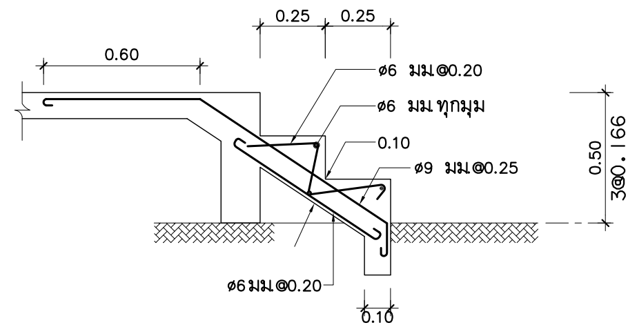
STX มาตราส่วน 1:20
