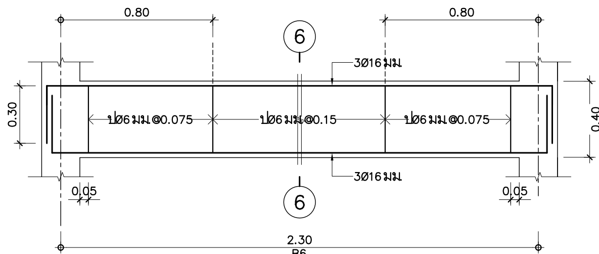
B6 มาตราส่วน 1:20
