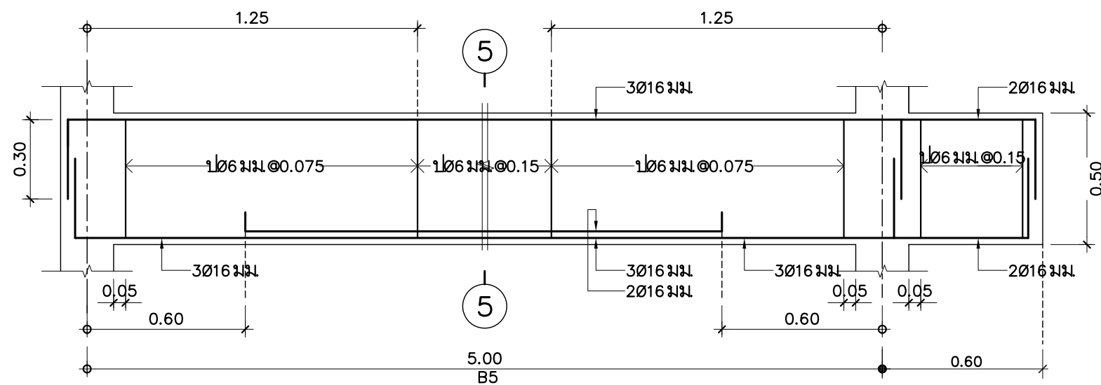
B5 มาตราส่วน 1:20
