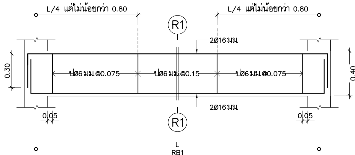
RB1 มาตราส่วน 1:20
