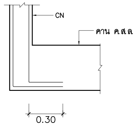
รอยต่อเสา CN กับ คาน ค.ส.ล. มาตราส่วน 1:20
