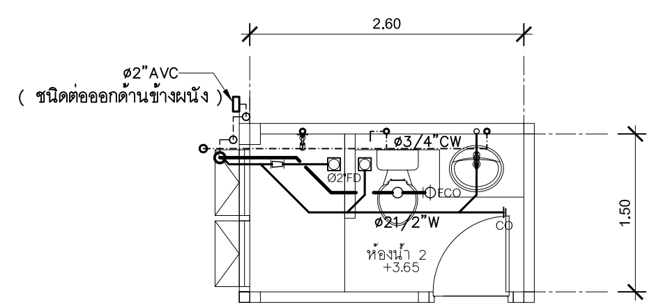
แปลนระบบสุขาภิบาลห้องน้ำ 2 มาตราส่วน 1 : 50 ( ท่อประปาเดินใต้พื้น )
