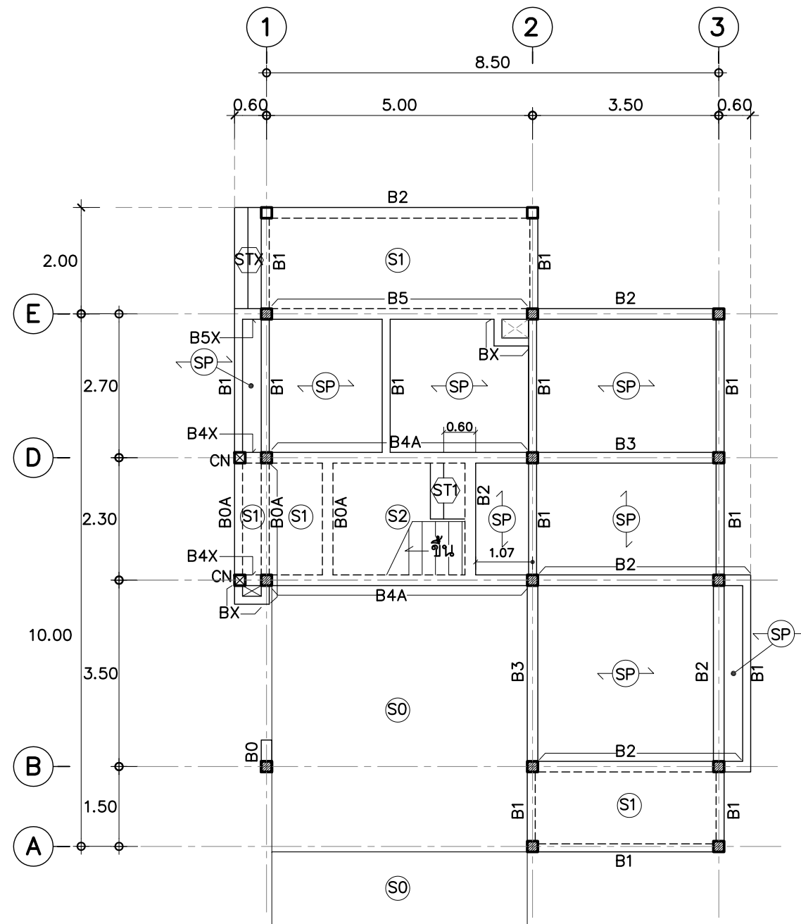
แปลนคาน, พื้นชั้น 1 มาตราส่วน 1 : 100
