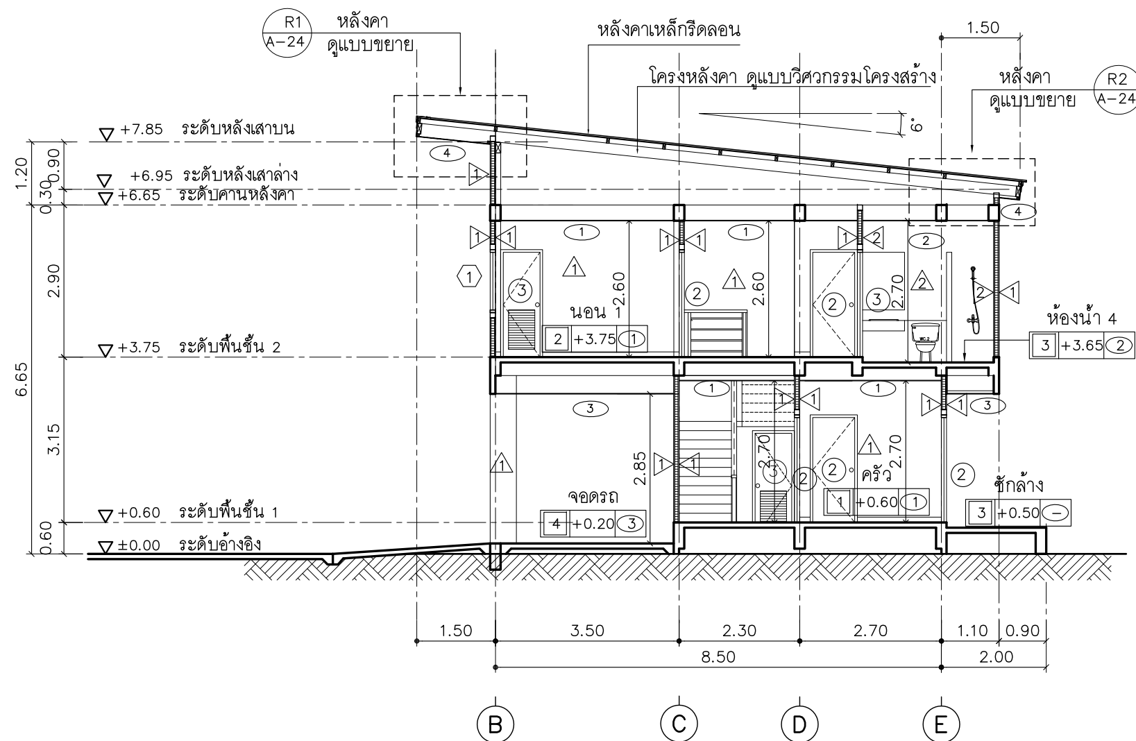
รูปตัด 3 มาตราส่วน
