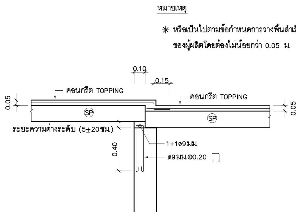
ลักษณะการหล่อพื้นเสริมกรณีพิเศษช่องว่างที่คานริม มาตราส่วน 1: 20
