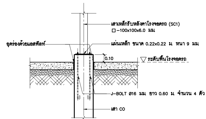
แบบขยายฐานรับเสาเหล็กรับหลังคาโรงจอดรถ 1:25
