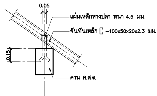
แบบขยายการยึดจันทันเหล็กกับคาน ค.ส.ล. 1:25
