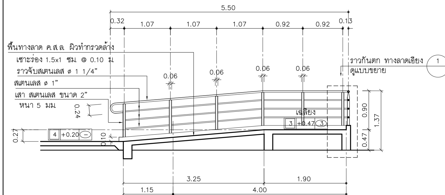
รูปตัดทางลาดเอียง R.1
