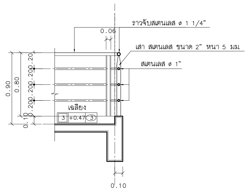
แบบขยายราวกันตก
