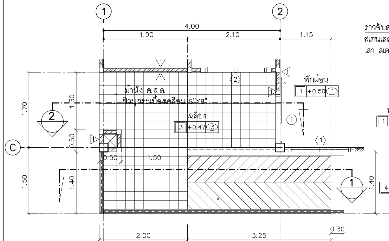
แปลนทางลาดเอียง R.1
