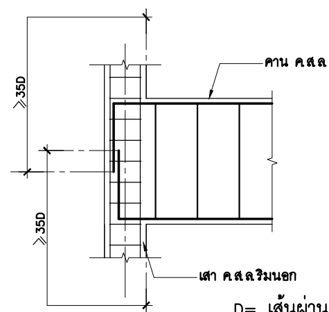
แบบขยายการฝังเหล็กเสริมคาน ค.ส.ล. เข้าเสา ค.ส.ล. 1:25
