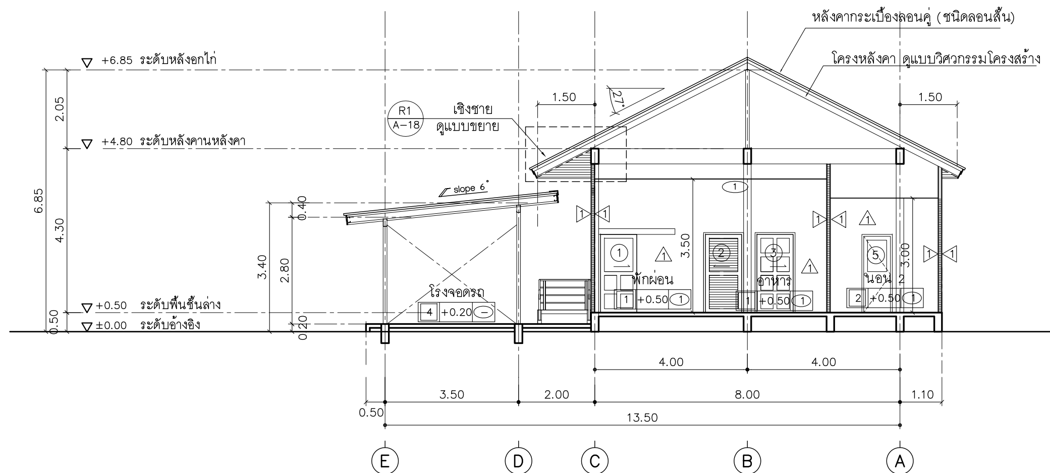
รูปตัด 2
