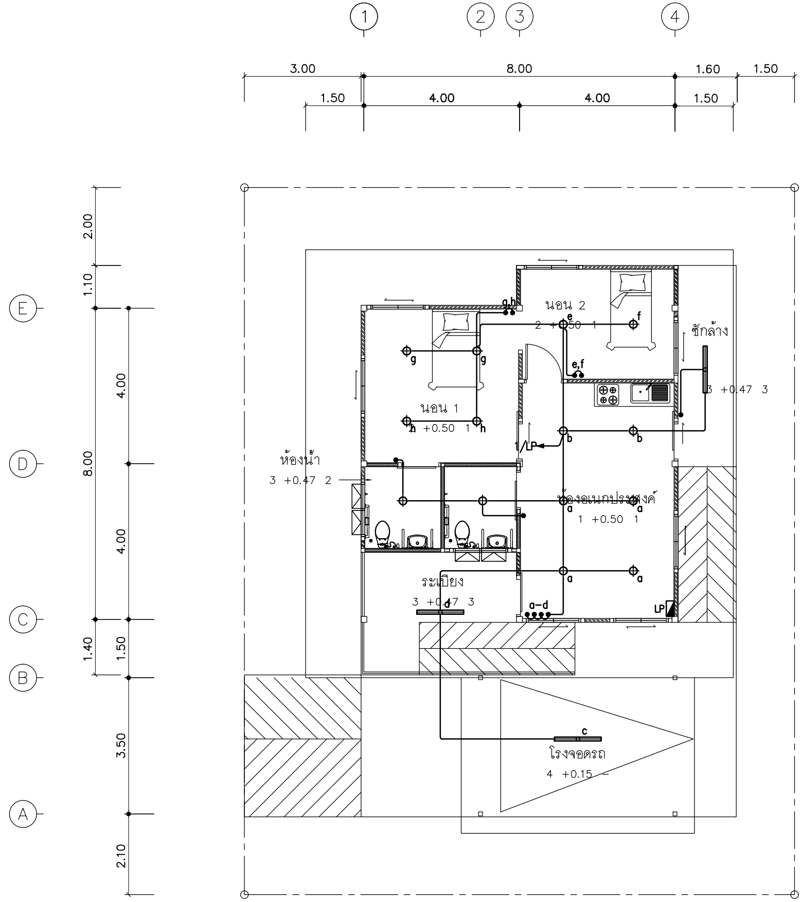
แปลนไฟฟ้าแสงสว่าง 1:100
