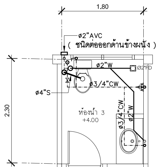
แปลนระบบสุขาภิบาลห้องน้ำ 3 มาตราส่วน 1 : 50 ( ท่อประปาเดินใต้พื้น )
