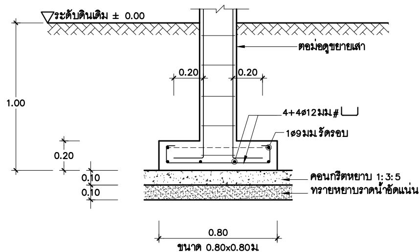
F0.80x0.80 มาตราส่วน 1: 25
