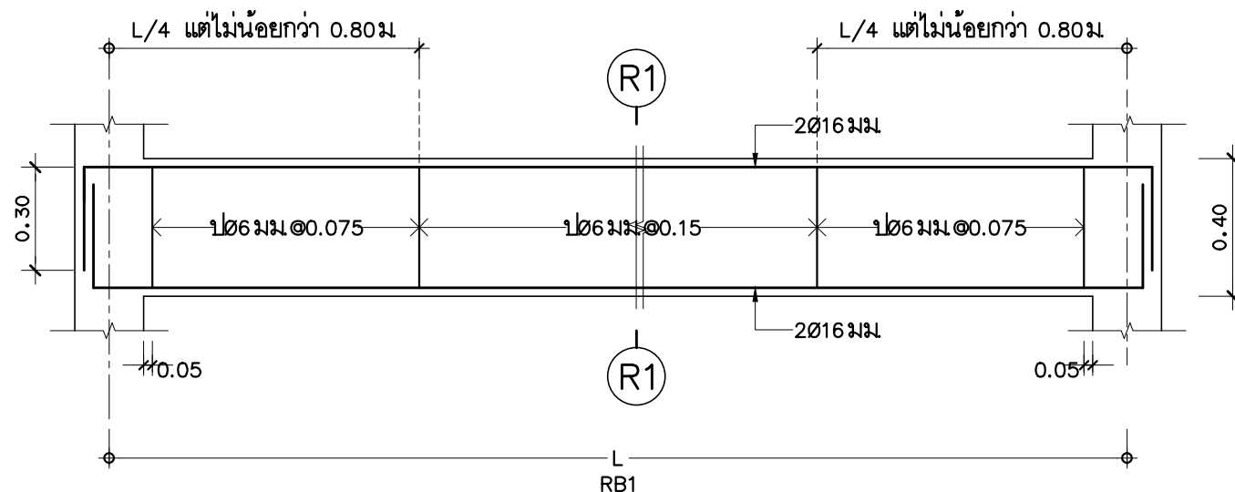
RB1 มาตราส่วน 1:20
