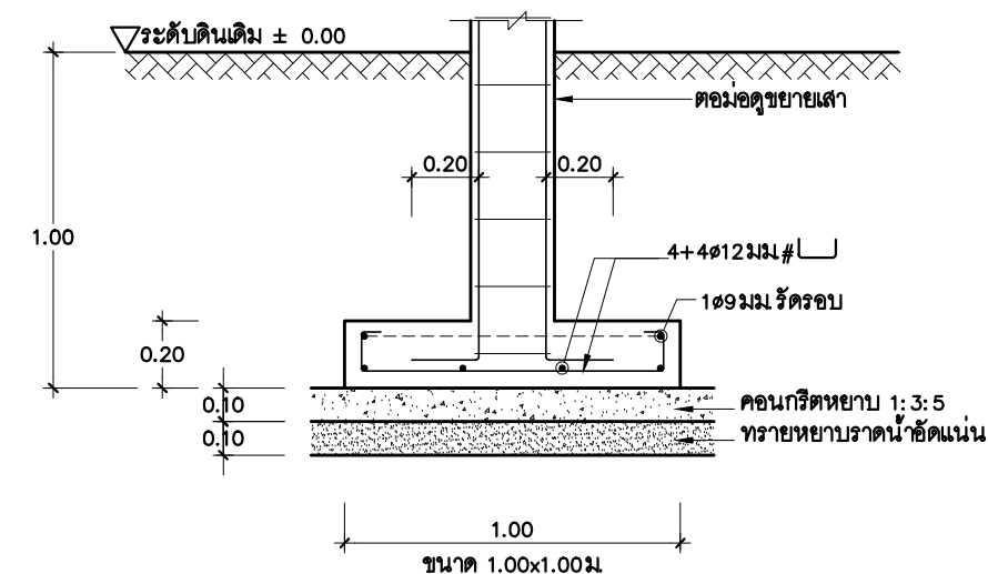
F1.00x1.00 มาตราส่วน 1: 25
