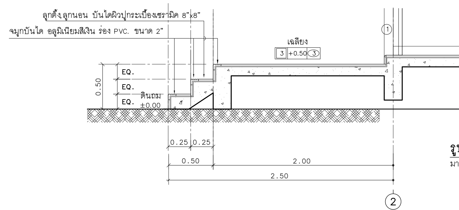
แปลนบันได ST.2 มาตราส่วน 1:25
