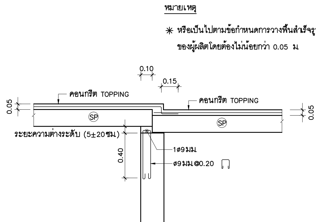
กรณียกระดัดพื้นสำเร็จต่างระดับกัน มาตราส่วน 1: 20
