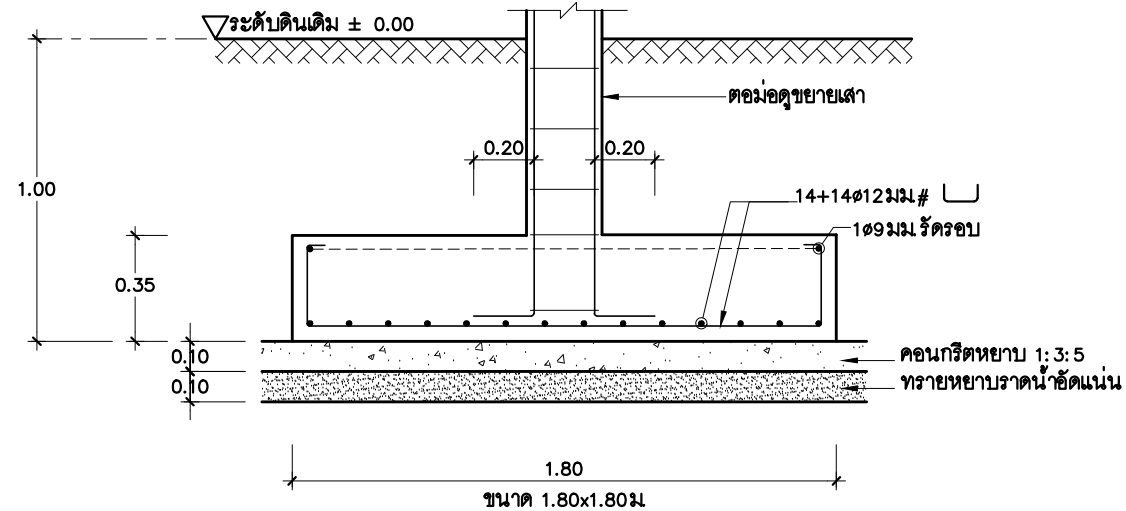
F1.80x1.80 มาตราส่วน 1: 25
