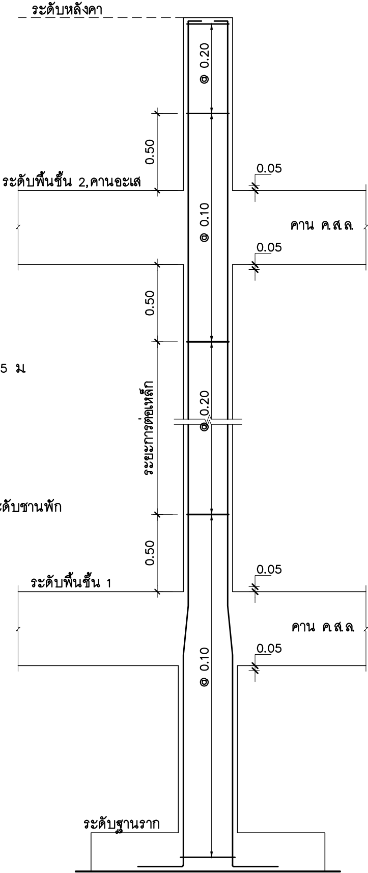
รายละเอียดการเสริมเหล็กปลอกในเสา
