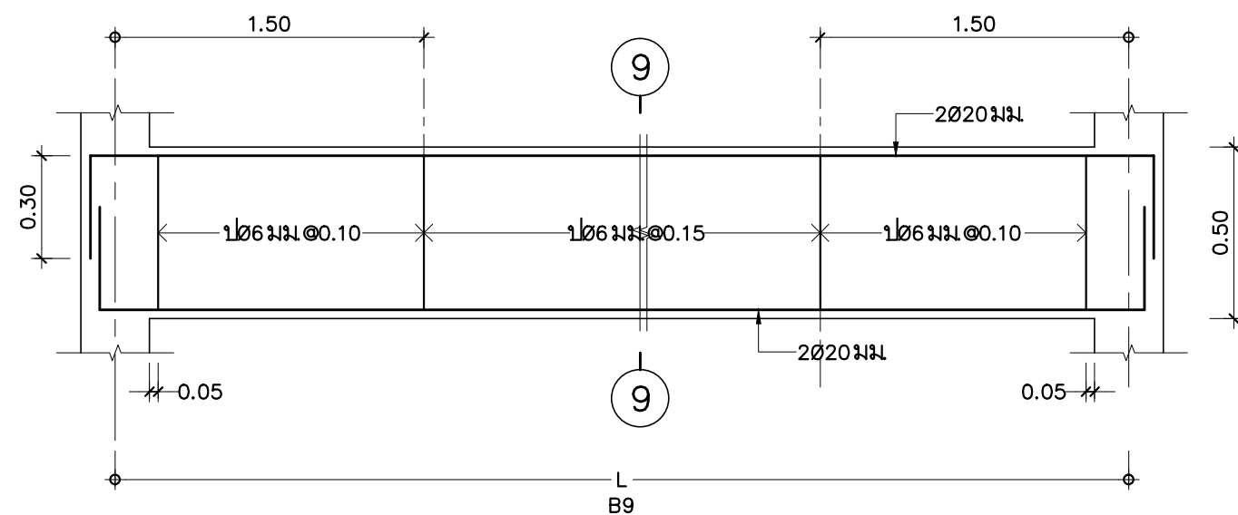
B9 มาตราส่วน 1: 20
