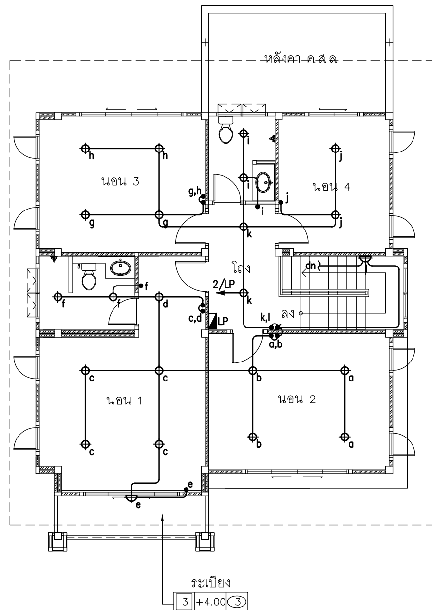
แปลนไฟฟ้าแสงสว่าง ชั้นบน 1 : 100
