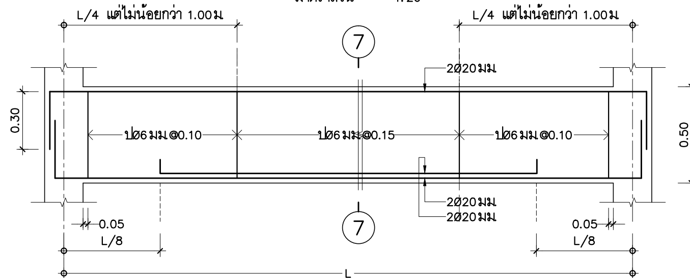
B7 มาตราส่วน 1: 20
