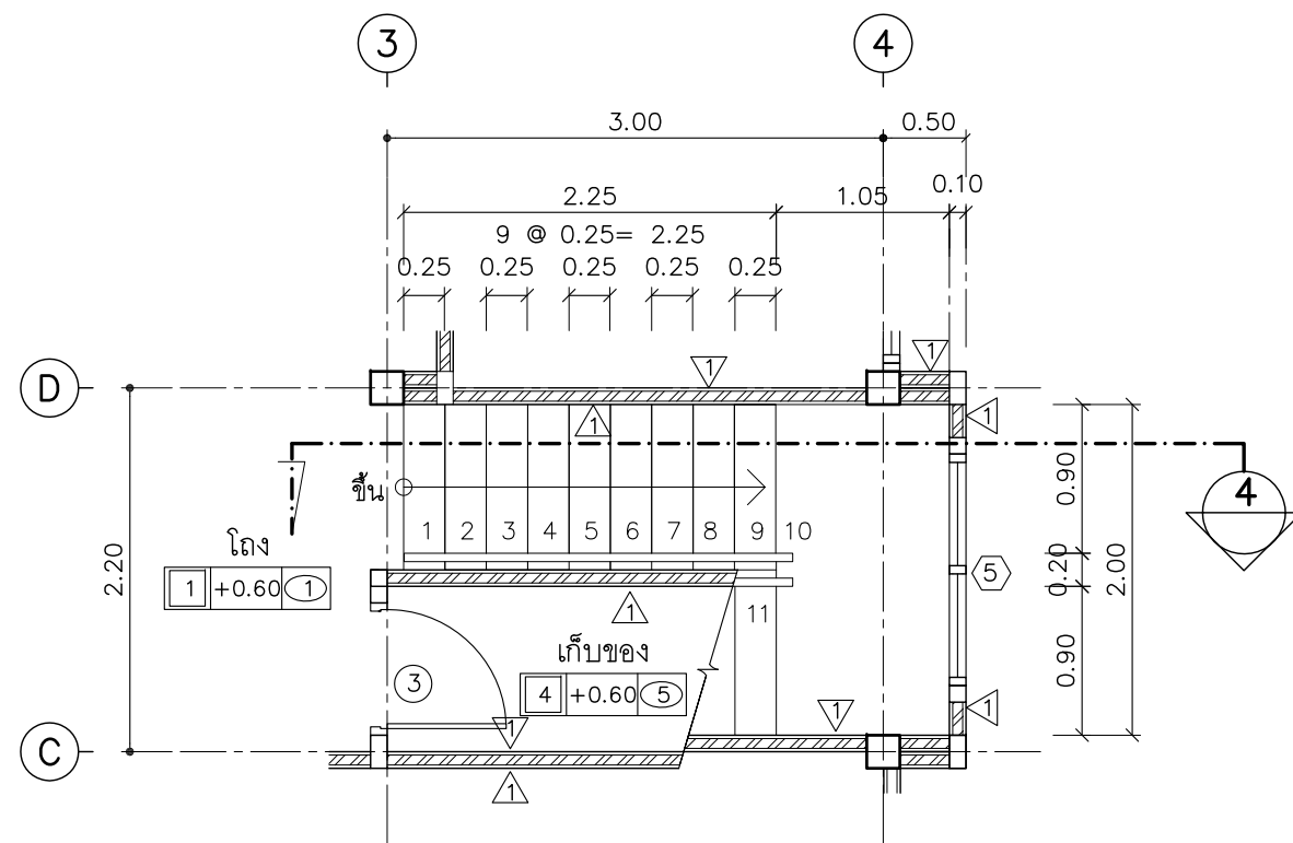
แปลนชั้น 1 บ้านได ST.3
