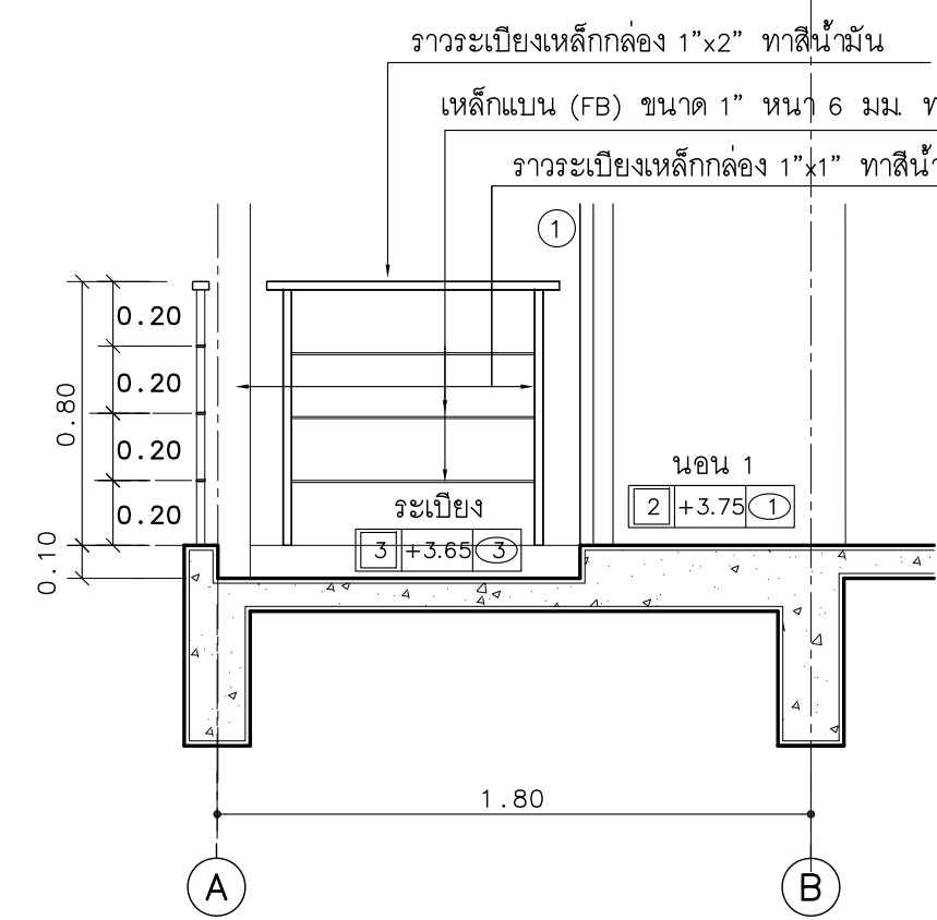
แบบขยาย รูปตัดราวกันตก มาตราส่วน 1: 25
