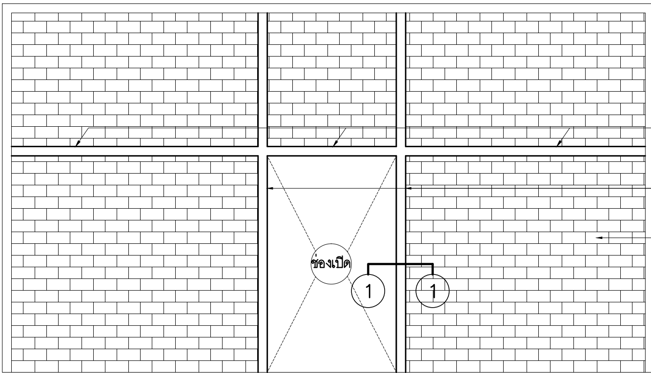
รายละเอียดการก่อสร้างเสาค้ำและคานทับหลังคอนกรีตบริเวณช่องเปิด
