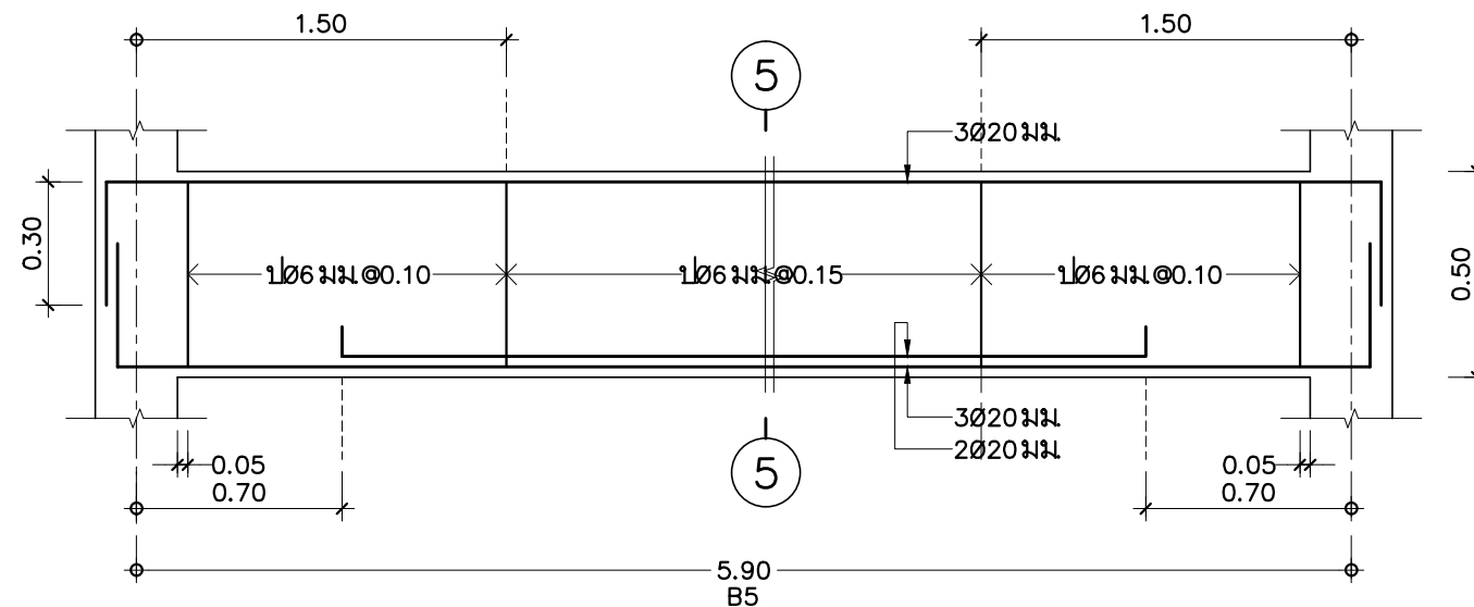
B5 มาตราส่วน 1: 20
