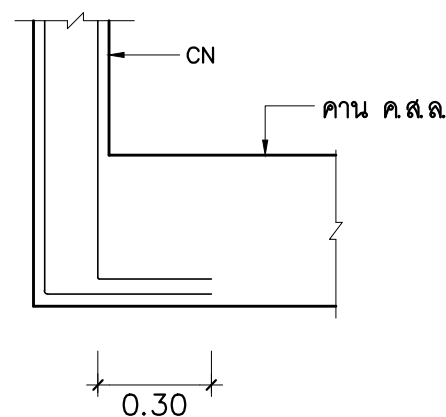
รอยต่อเสา CN กับ คาน ค.ส.ล. มาตราส่วน 1:20
