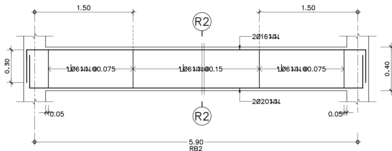
RB2 มาตราส่วน 1:20
