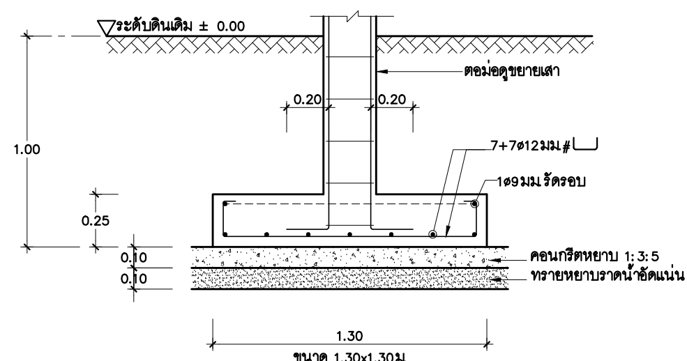
F1.30x1.30 มาตราส่วน 1: 25
