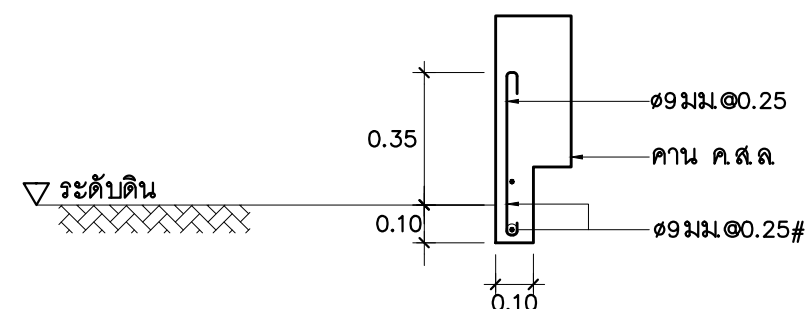
แบบขยายคาน ค.ส.ล. รอบอาคาร มาตราส่วน 1:20
