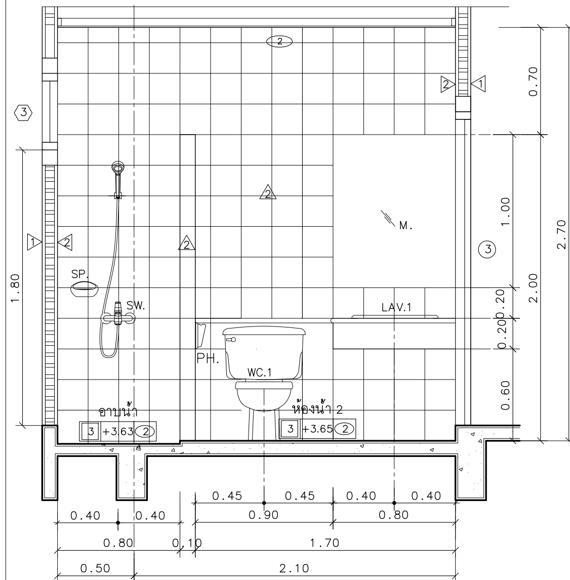
รูปตัดห้องน้ำ WC.2
