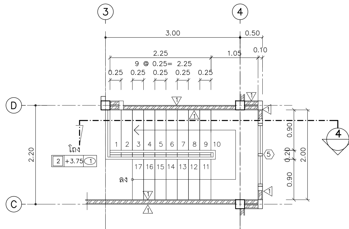
แปลนชั้น 2 บ้านได ST.3
