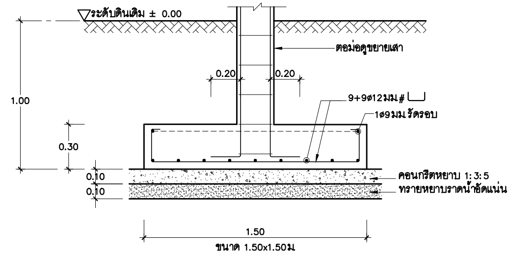
F1.50x1.50 มาตราส่วน 1: 25
