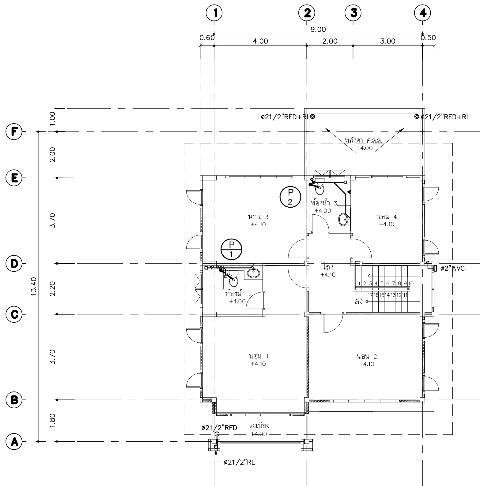
แปลนระบบสุขาภิบาลพื้นที่ชั้นบน มาตรฐาน 1 : 100
