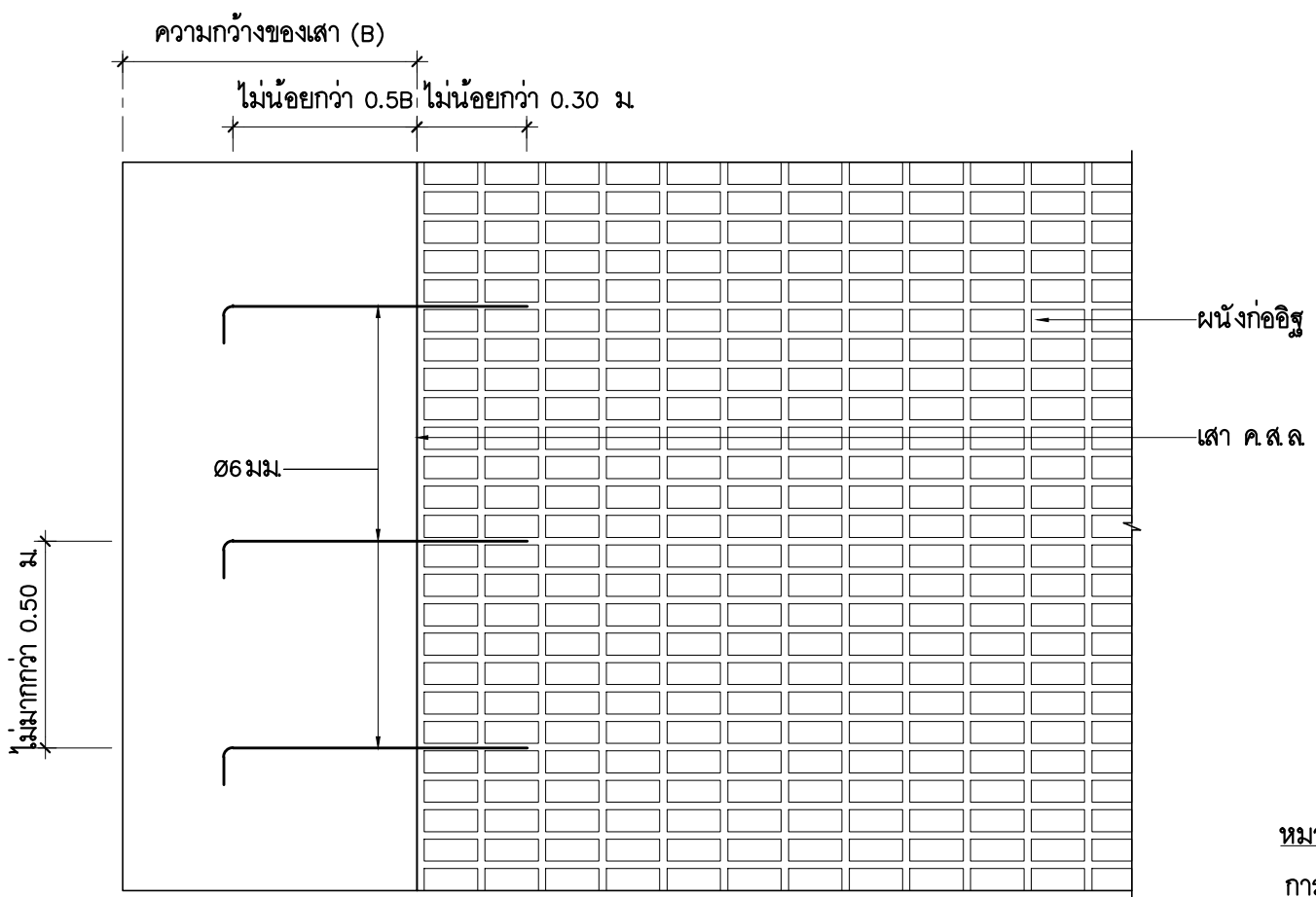
รายละเอียดการเสียบเหล็กหนวดกุ้ง
